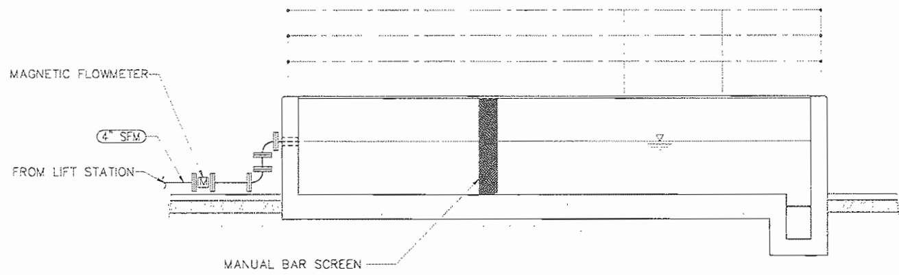
SECTION 2 SCALE: 1/2" = 1'-0"
